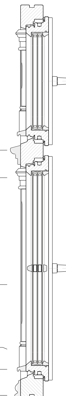
Fenster Vertikalschnitt
